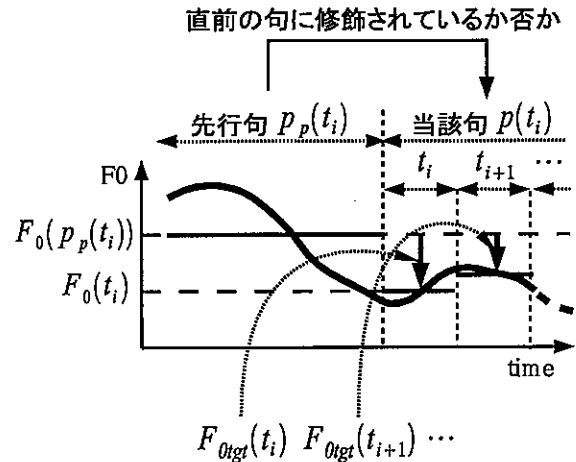
図 3: ターゲット特徴量の抽出
